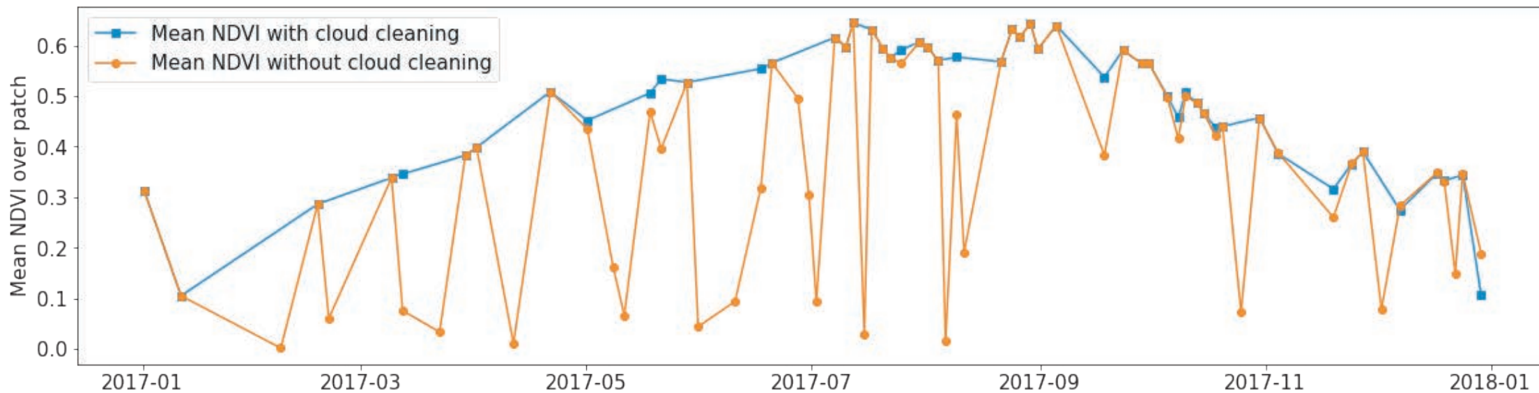
NDVI
